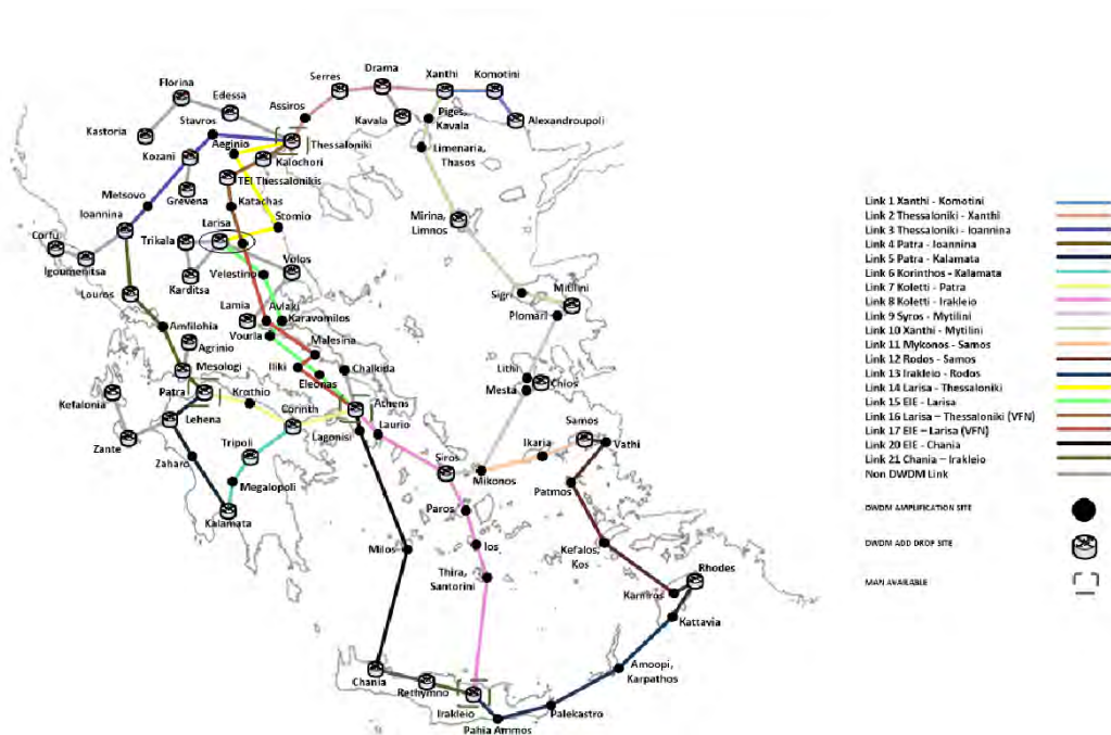
Εικόνα 7 Δίκτυο Οπτικών Ινών ΕΔΕΤ (WAN)
