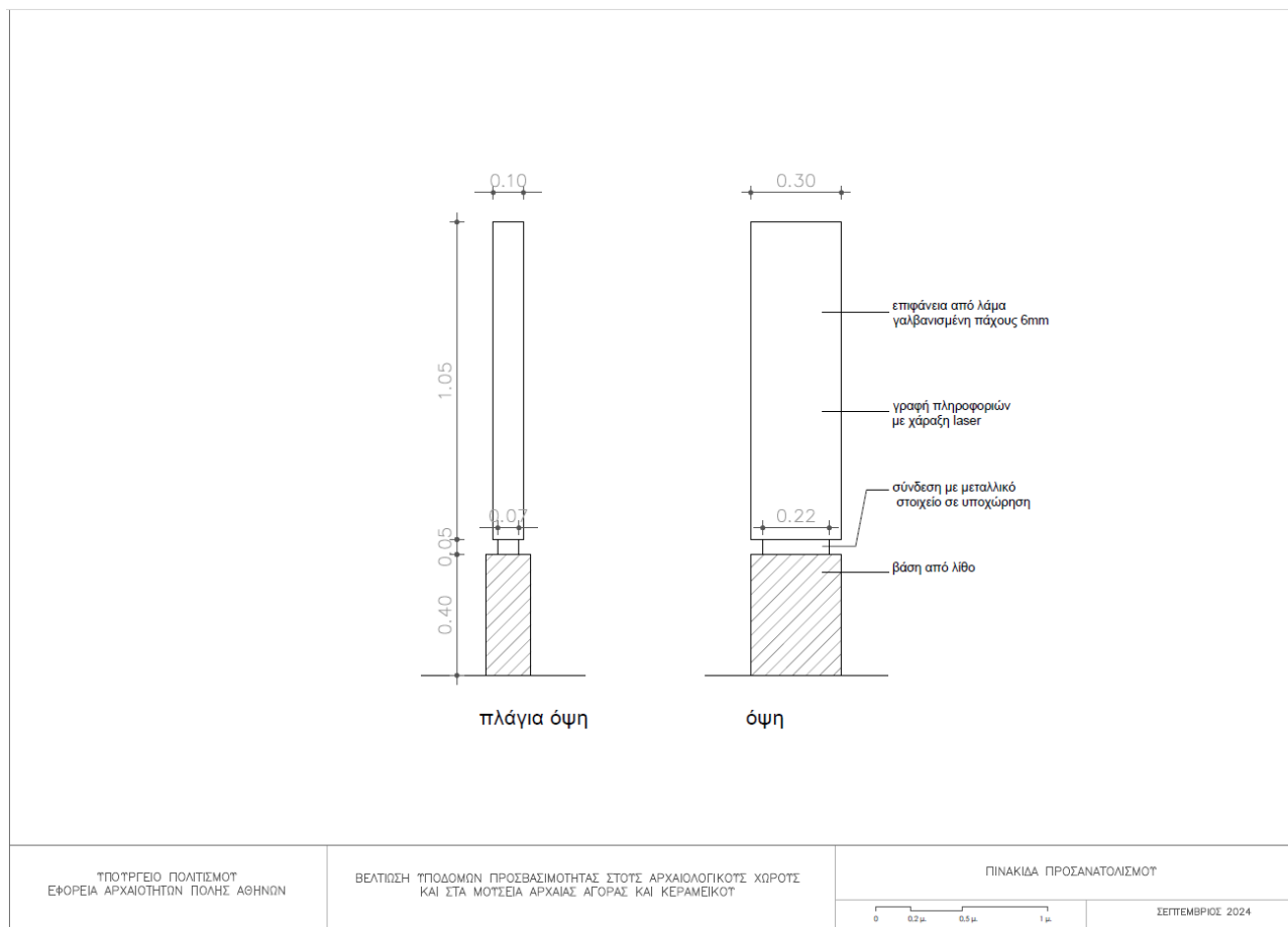
Σχ. 1 Πινακίδα προσανατολισμού
