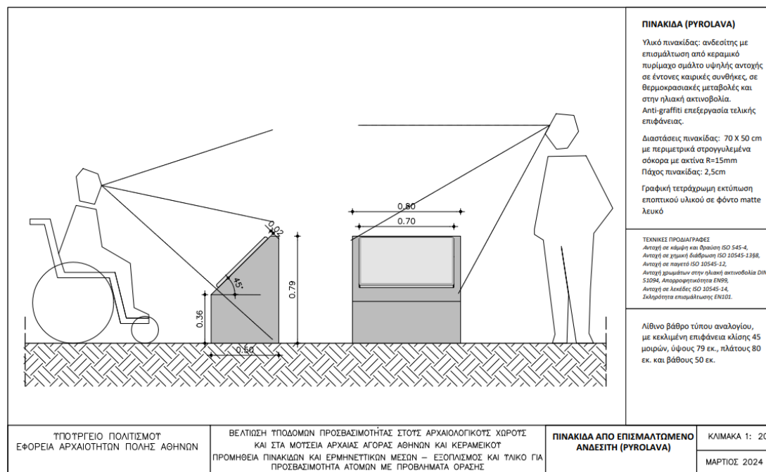
Σχ. 3 Πινακίδα Ρυγολάνα αναλόγιο επί εδάφους
