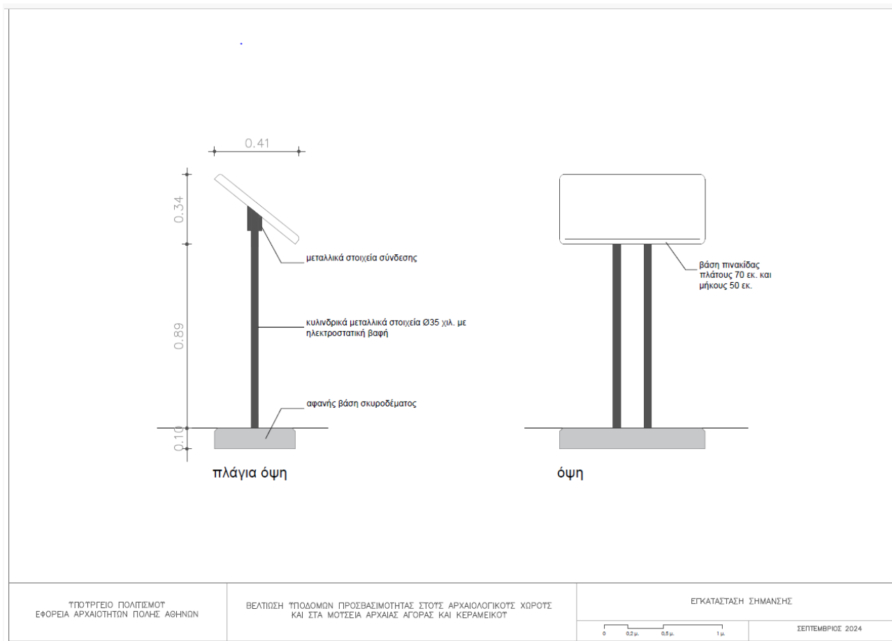
Σχ. 4 Ειδική πινακίδα Braille-ανάγλυφης κάτοψης
