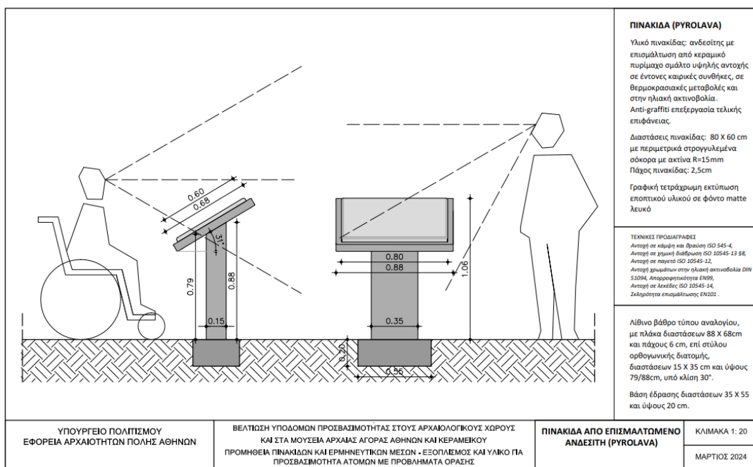
Σχ. 2 Πινακίδα Ρυγολάνα αναλόγιο με πόδι
