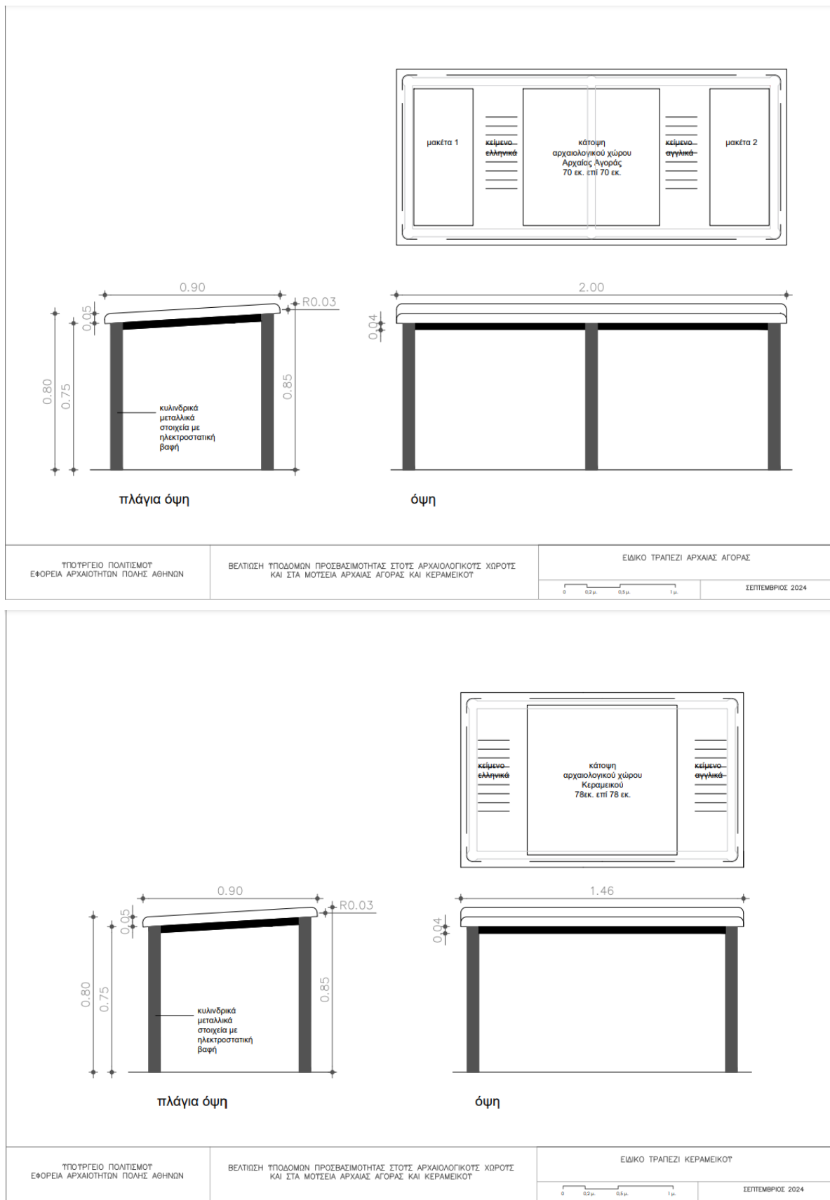
Σχ. 5 Ενδεικτικό σχέδιο τραπεζιού μακέτας και απτικού χάρτη
