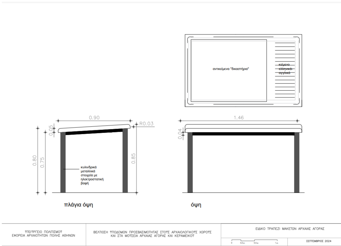
Σχ. 6. Ενδεικτικό σχέδιο τραπεζιού απτικών εκθεμάτων
